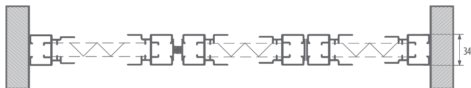
Sección horizontal 3 hojas
