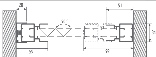
Sección horizontal 1 hoja
