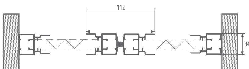
Sección horizontal 2 hojas
