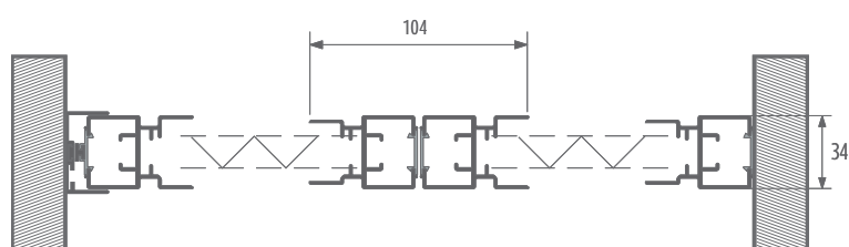
Sección horizontal 2 hojas para prolongar
