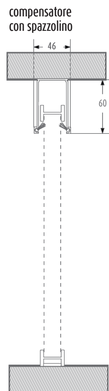
Sección vertical
